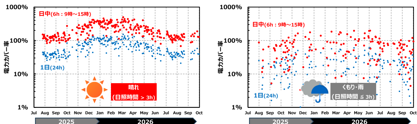
図 3. 晴れの日と、くもり・雨の日における日別電力カバー率の推移。 (2025 年 7 月 25 日～2026 年 9 月 30 日の実績データをプロット)
