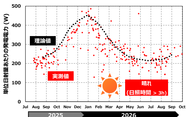
図 6. 気象データから算出した、晴れの日における単位日射量当たりの発電電力の理論値と実測値。
