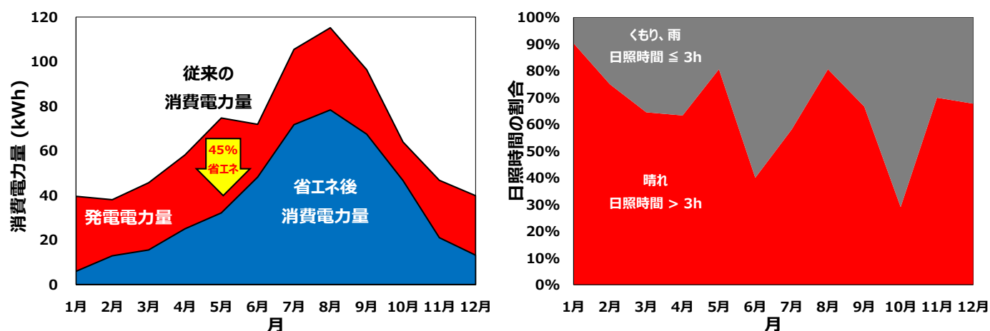
図 2. 月別発電電力量と消費電力量の推移および晴れの日割合。 (2025 年 8 月 1 日～2026 年 7 月 31 日の実績データより算出)
