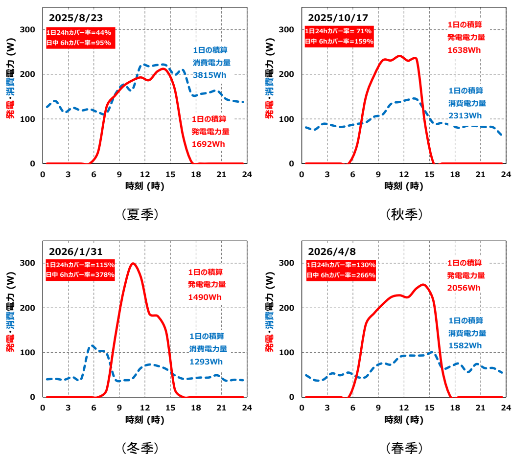
図 5. 各季節における、代表的な晴れの日の時間別発電電力および消費電力の推移。
