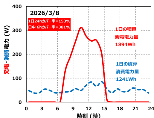
図 4. 最も電力カバー率の高い日の、時間別発電電力および消費電力の推移。
