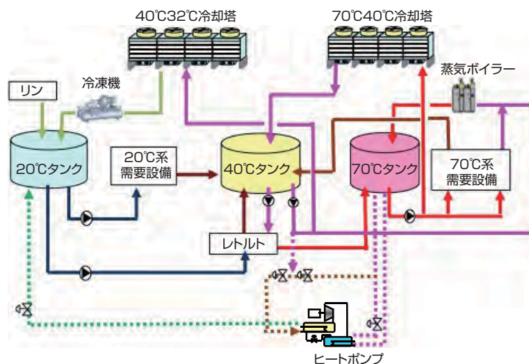
ヒートポンプと循環水システムの概要
